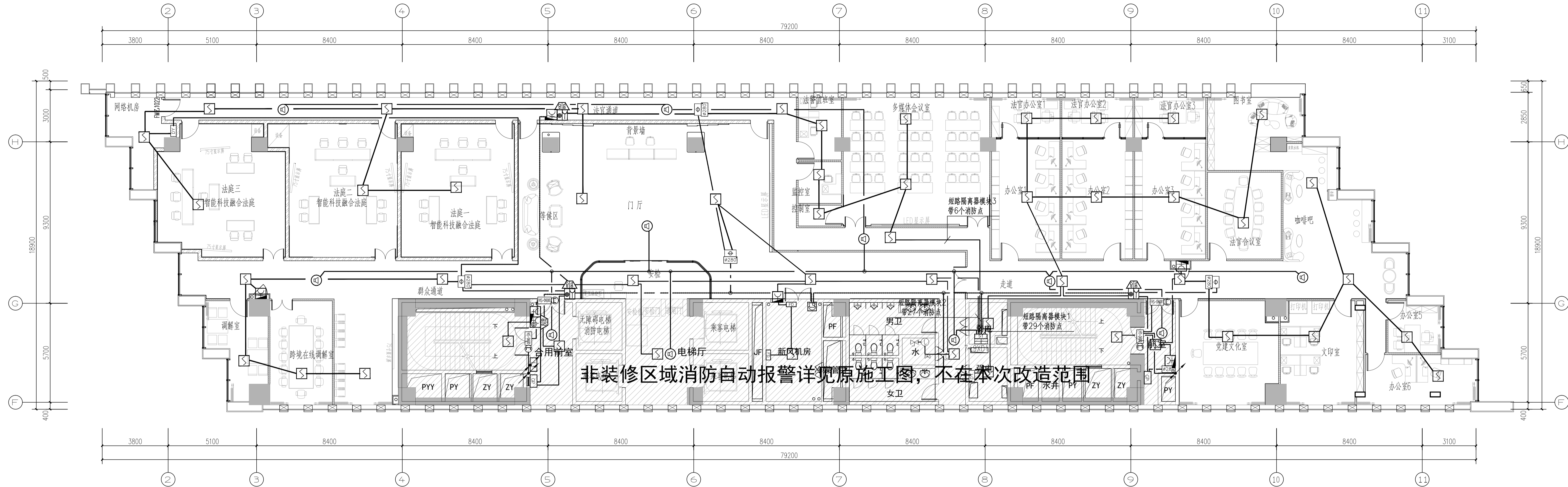
八层消防自动报警平面图 1:100
